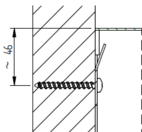
SCHÉMA ZAVĚŠENÍ
